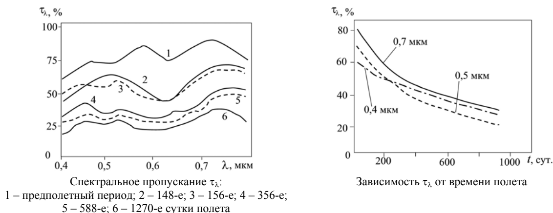
Рис. 4. Результаты исследования оптических характеристик: а) иллюминатора ОНС «Салют-4»; б) иллюминатора ОНС «Салют-6»
